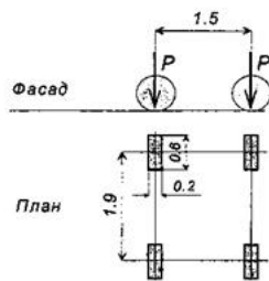
Рисунок 18.1 - Схема навантаження тандема АК
