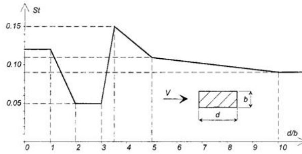
Рисунок Л.2.1 - Значення числа Струхала для прямокутного тіла
