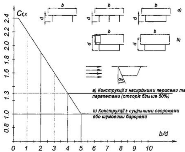
Рисунок Л.1 - Графік зміни коефіцієнта C_{f,x}
