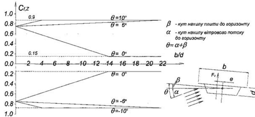
Рисунок Л.2 - Графік зміни коефіцієнта C_{fz}
