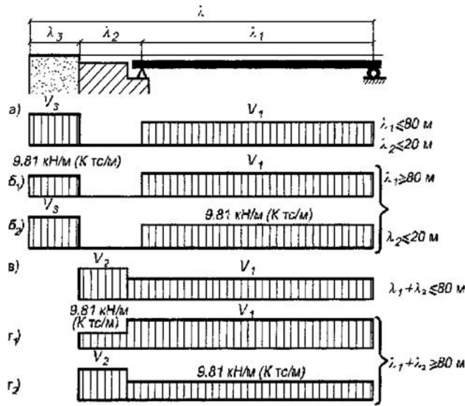
Рисунок Б.4 - Схема завантаження прогону одночасно з призмою обвалення або прогону зі стояном при розрахунку масивних стоянів мостів з розрізними балковими прогоновими будовами
