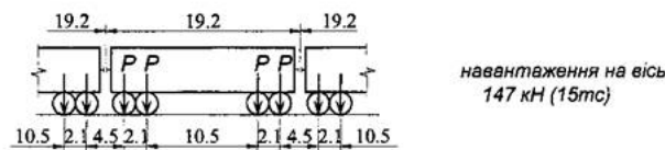
Рисунок 10.1 - Модель тимчасового навантаження потягу метрополітену
