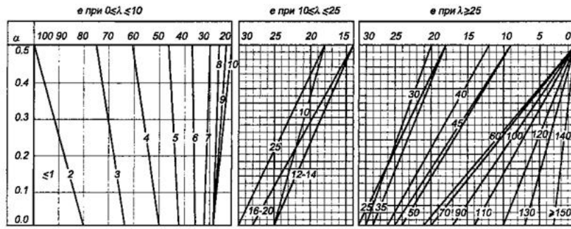
Рисунок Б.1 - Коэффициент e в зависимости от \lambda и \alpha (длина навантаження \lambda , м)
