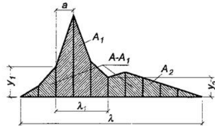
Рисунок Б.2 - Частина лінії впливу завдовжки \lambda_1 , що включає її вершину
