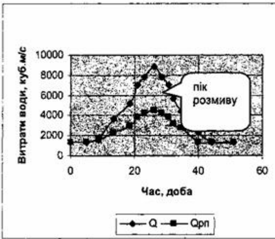
Рисунок Г.1 - Гідрографи загальної і руслової витрати
