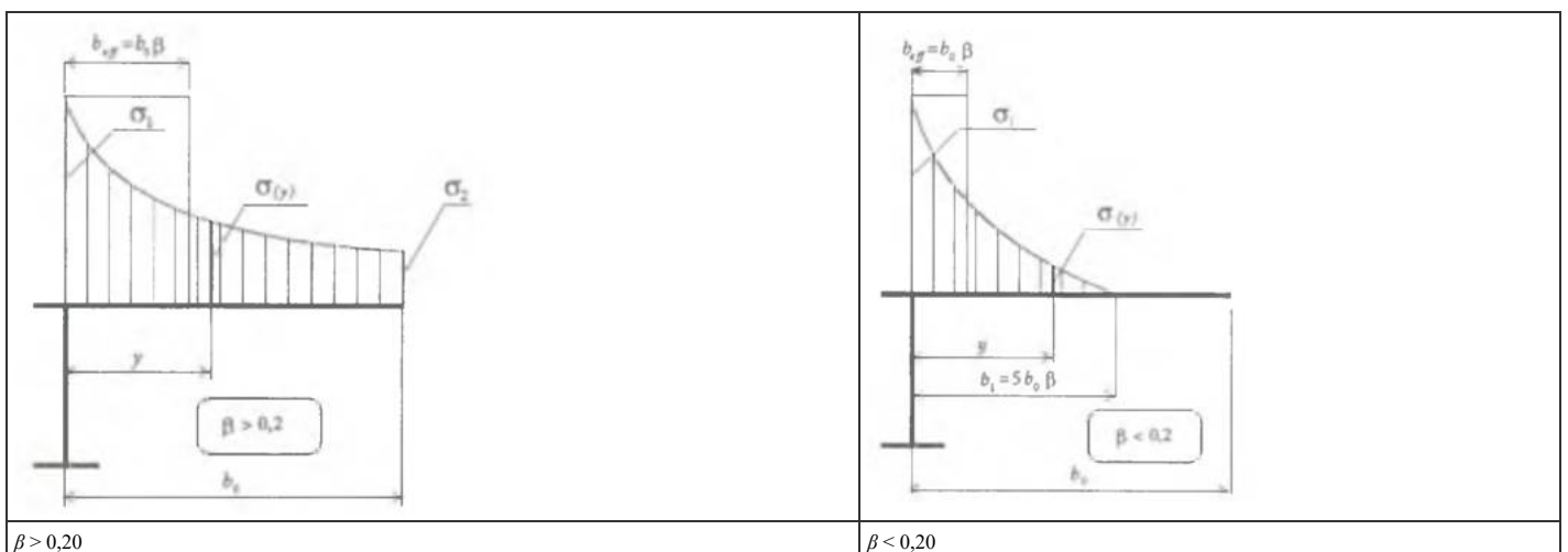
Таблиця Д.2 - Кількісна оцінка нерівномірності розподілу напружень
