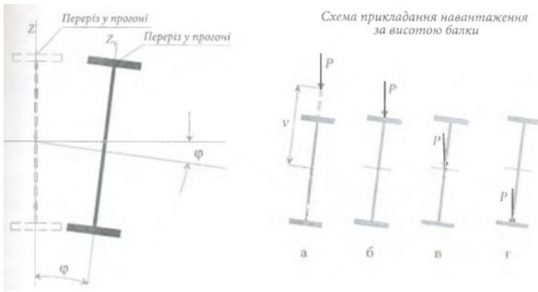
Рисунок И.1 - Поперечний переріз I-подібної зігнутої балки при згинально-крутній формі втрати стійкості
