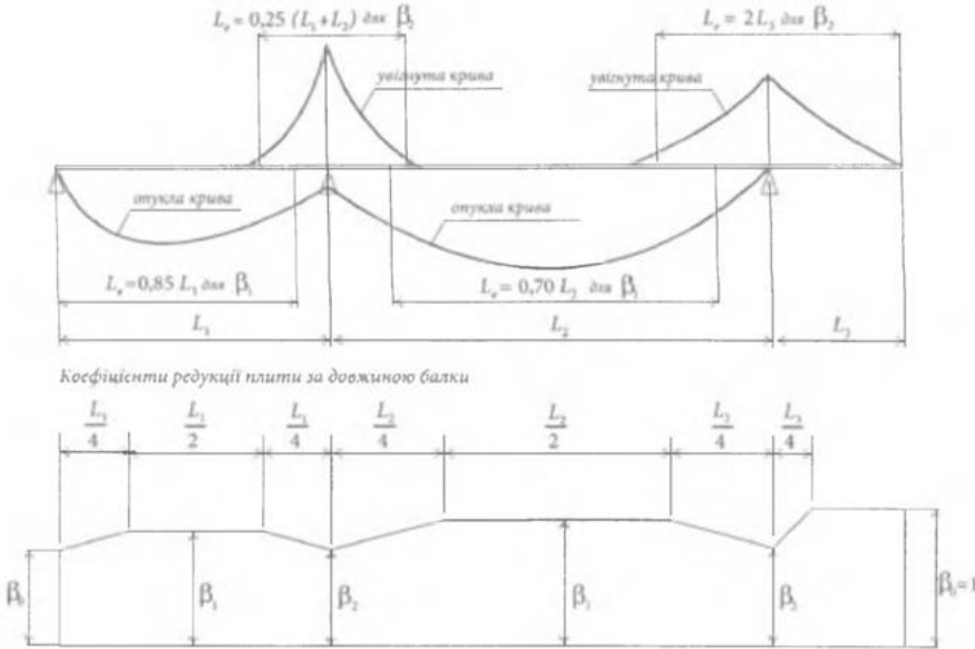
Рисунок Д.3 - Схема для визначення ефективної довжини прогону L_e .
