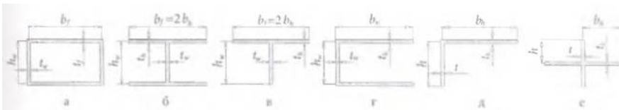
Рисунок 10.1 - Схеми розрахункових перерізів елементів, не підкріплених ребрами жорсткості
