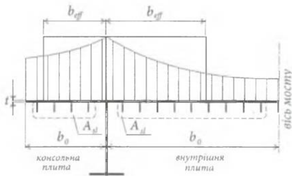
Рисунок Д.2 - Схема визначення коефіцієнта редукції для пружної роботи
