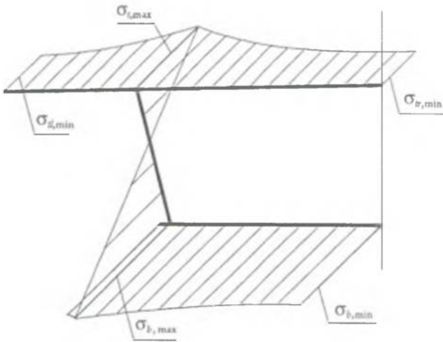
Рисунок Д.1 - Нерівномірність розподілу напружень у перерізі балки
