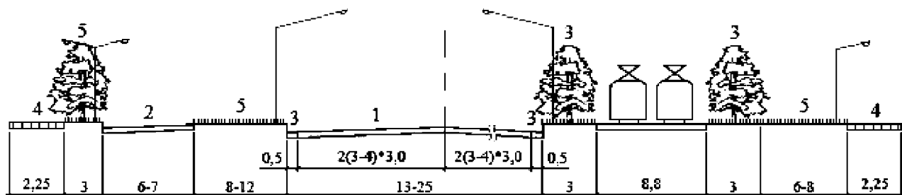
Магістральні вулиці загальноміського значення: I – безперервного руху; II, III – регульованого руху
