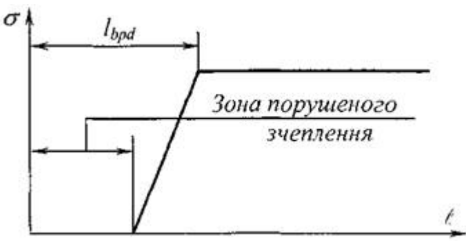
Рисунок 5.4 - Зона анкерування попередньо напруженої арматури, яка натягується на упори
