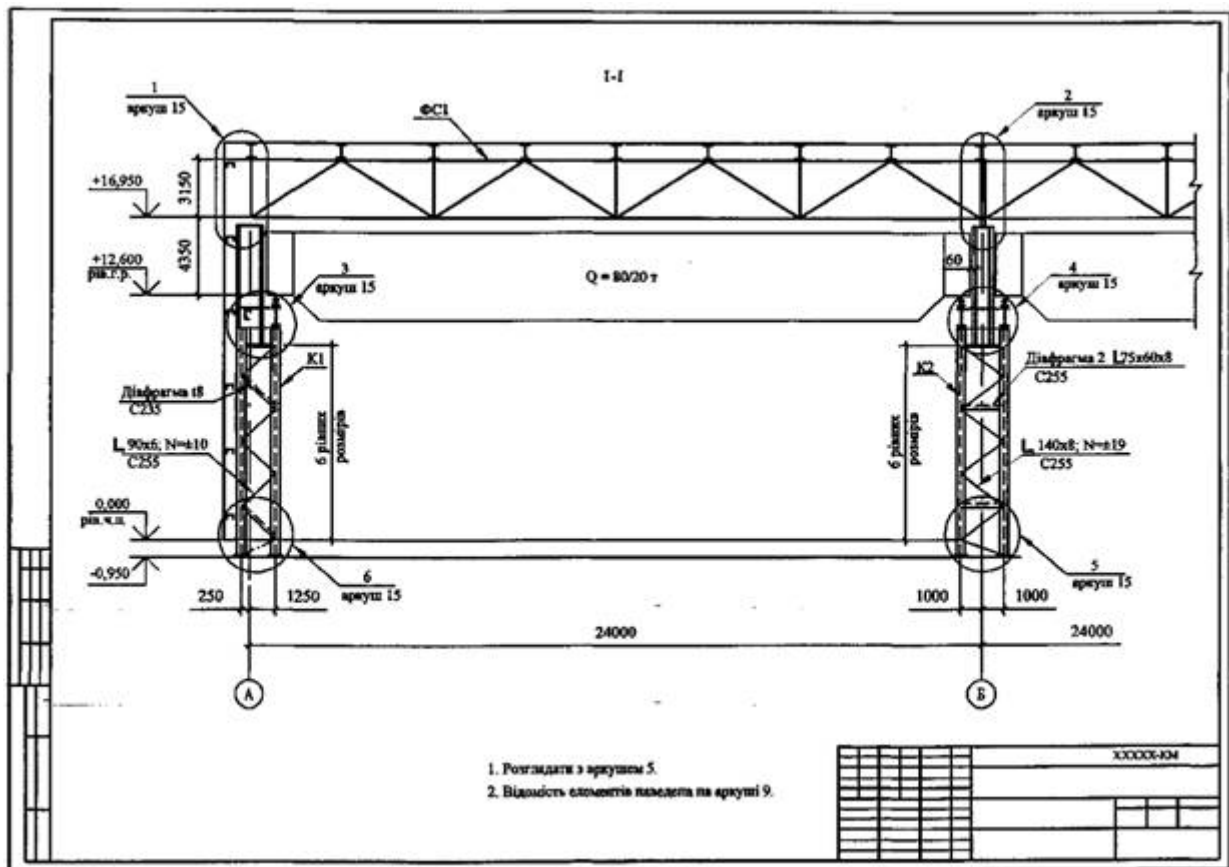
Рисунок Б.5 - Переріз 1-1
