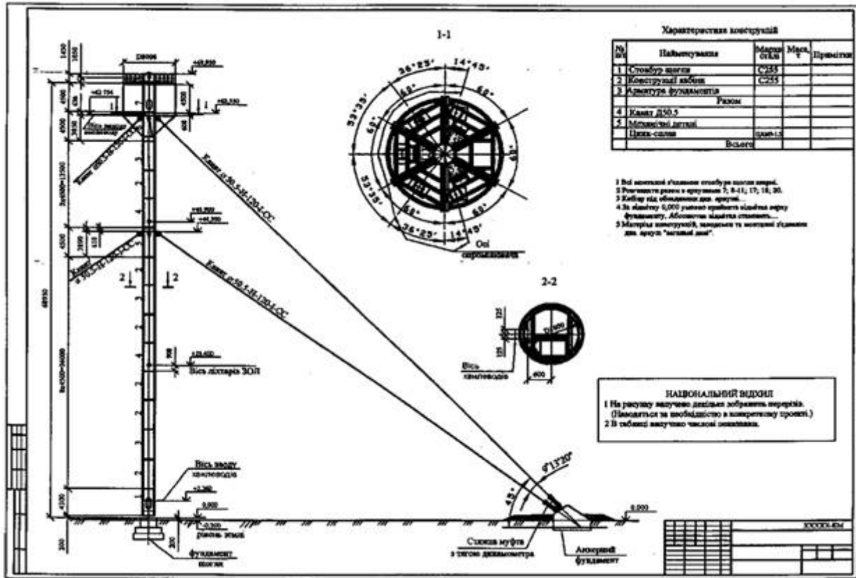
Рисунок Б.2 - Загальний вид шогли
