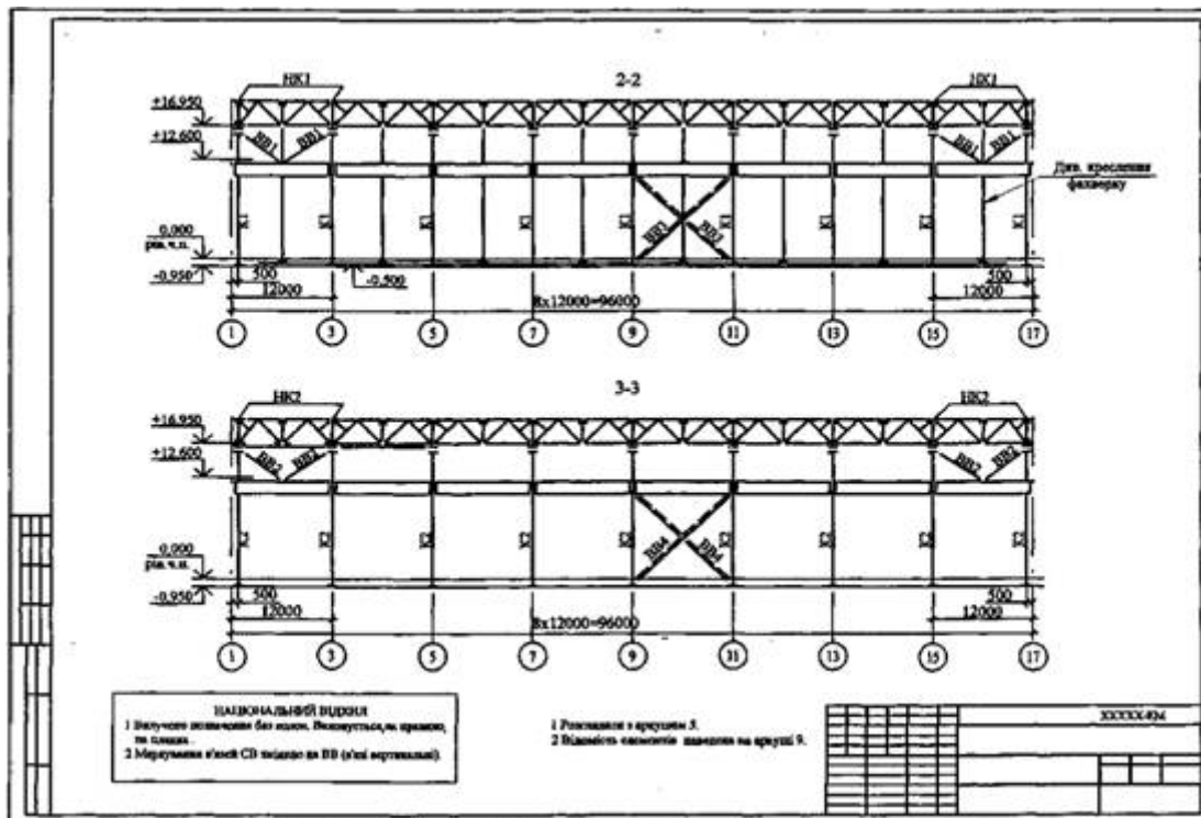
Рисунок Г.1 - Перерізи 2-2; 2-3
