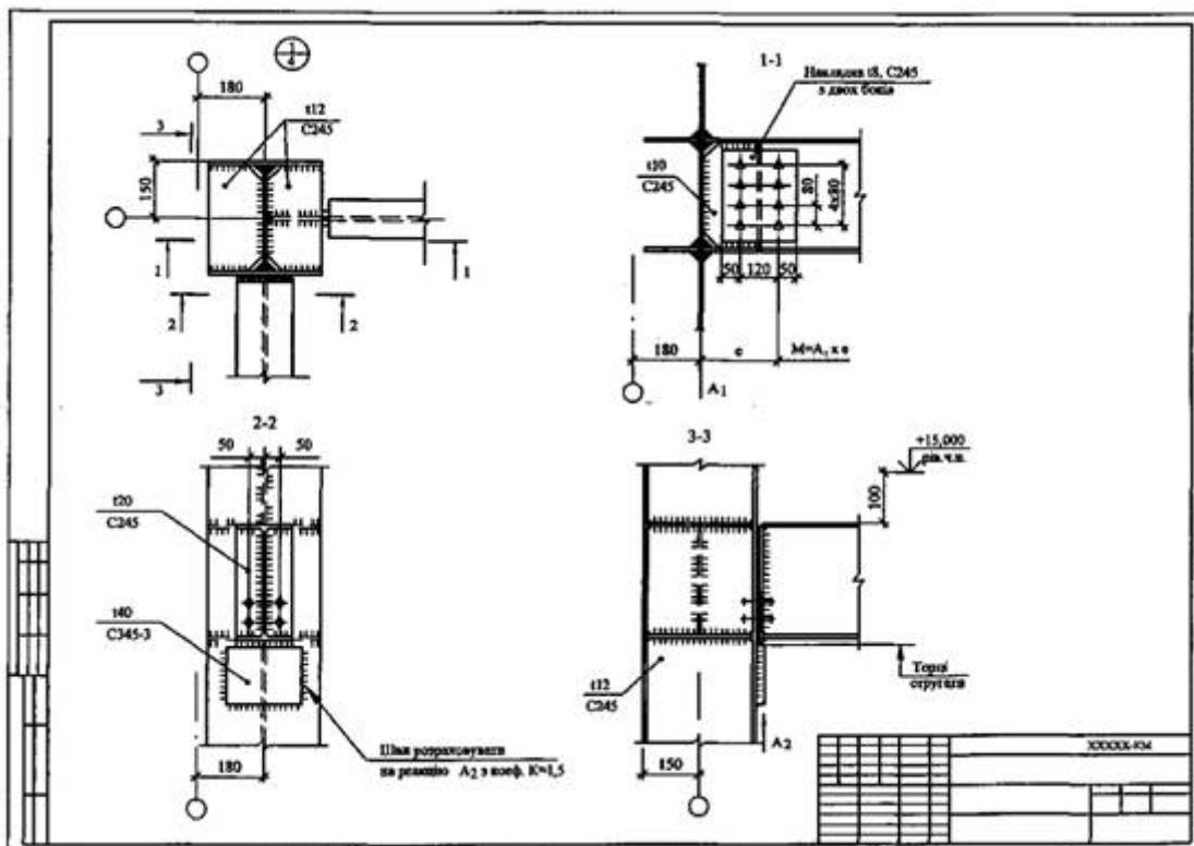
Рисунок Е.1 - Вузол 1
