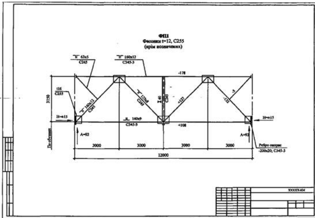
Рисунок Д.1 - Ферма підкрівля ФПІ
