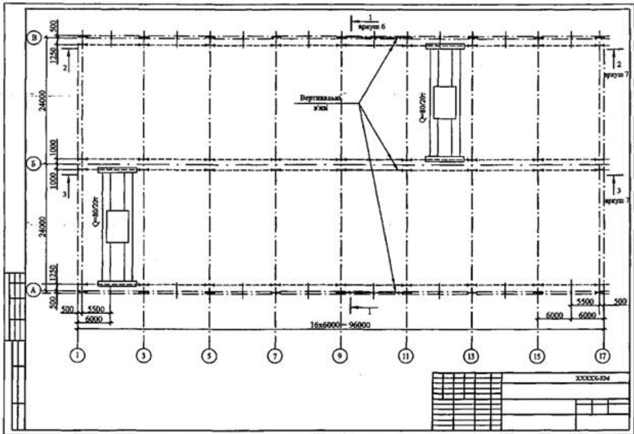
Рисунок Б.4 - Схема розташування колон на відмітці 0,000 м
