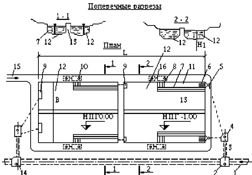
Рис. 2. Схема четырехсекционного пруда-отстойника:
