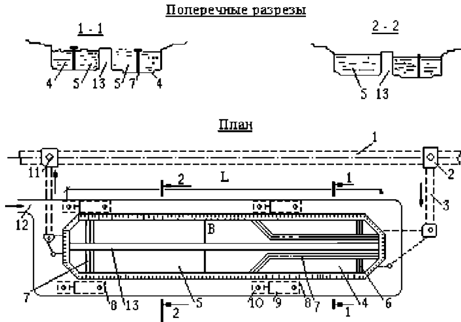
Рис. 1. Схема двухсекционного пруда-отстойника:
