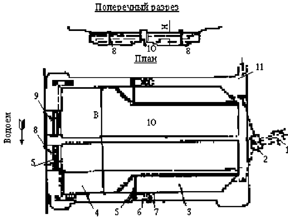
Рис. 5. Схема пруда-отстойника на сопряжении с водоемом:
