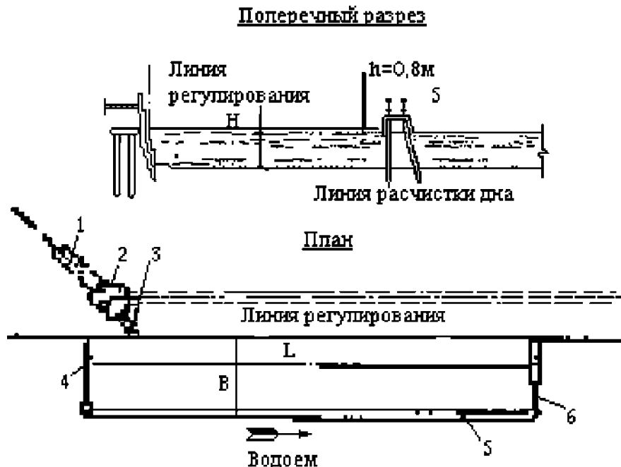
Рис. 6. Схема стационарного щитового заграждения:
