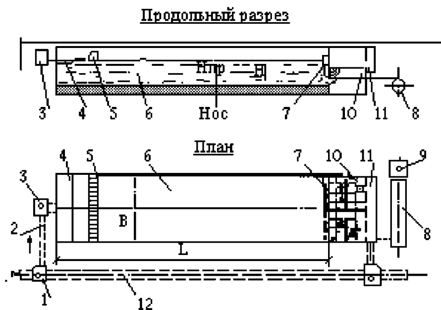
Рис. 7. Схема двухсекционного очистного сооружения закрытого типа:
